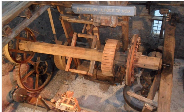
Le mécanisme du moulin à huile de noix
